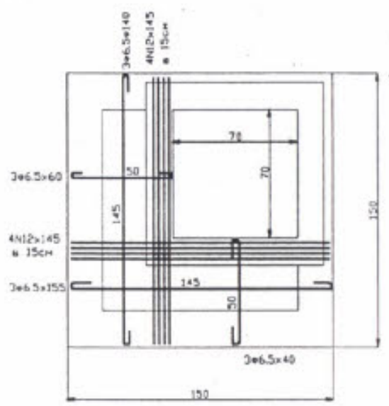
ПОКРИВНА ПЛОЧА
